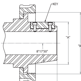
LONG TAPER
